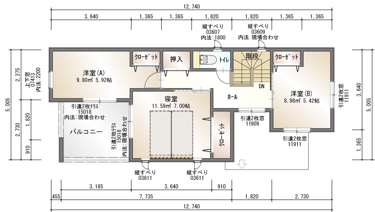
2階平面図
