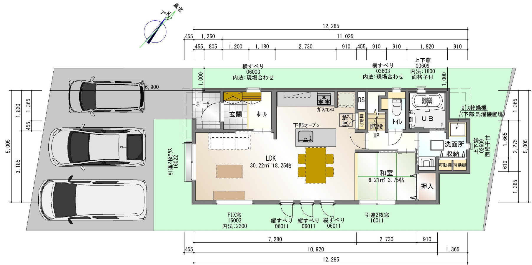
1階平面図
