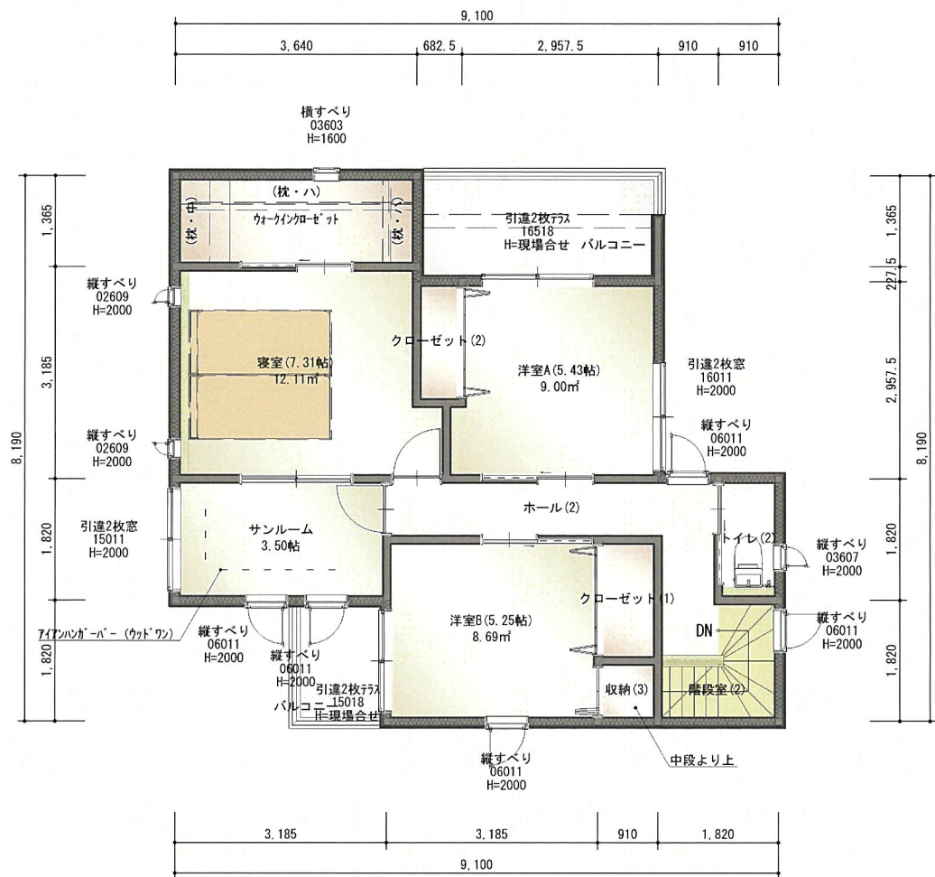
2 階平面図
