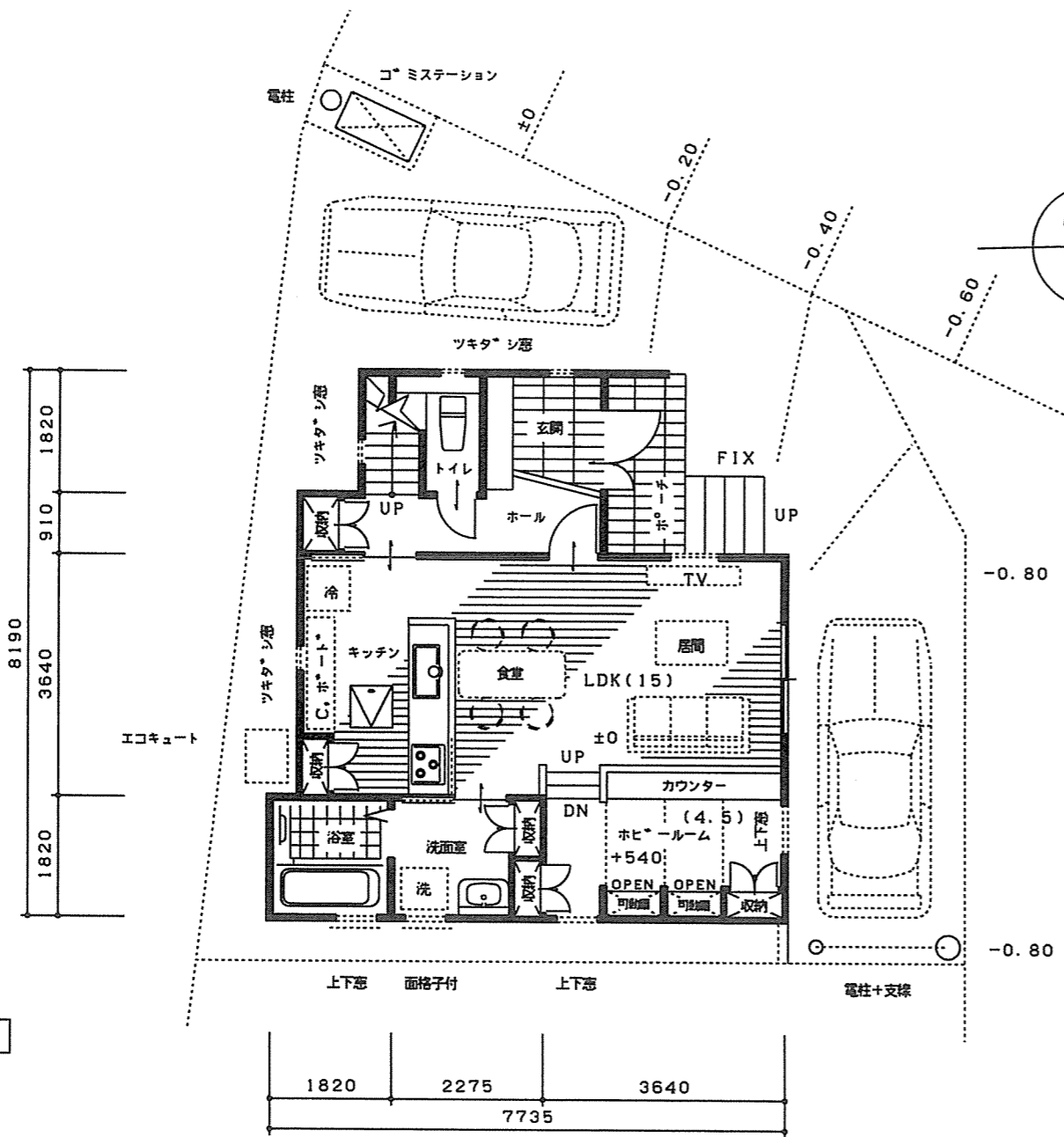
1階 平面図
