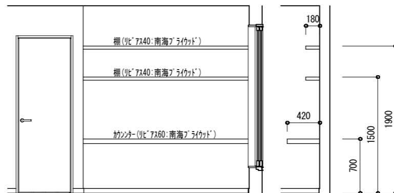
寝室展開図 1/50
