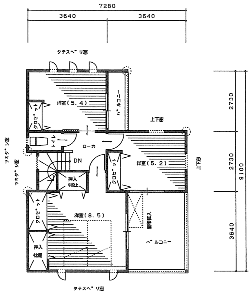
2階 平面図
