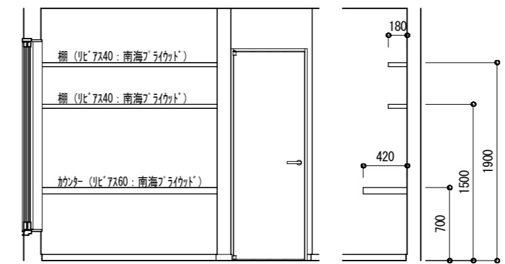
寝室カウンター展開図 1/50
