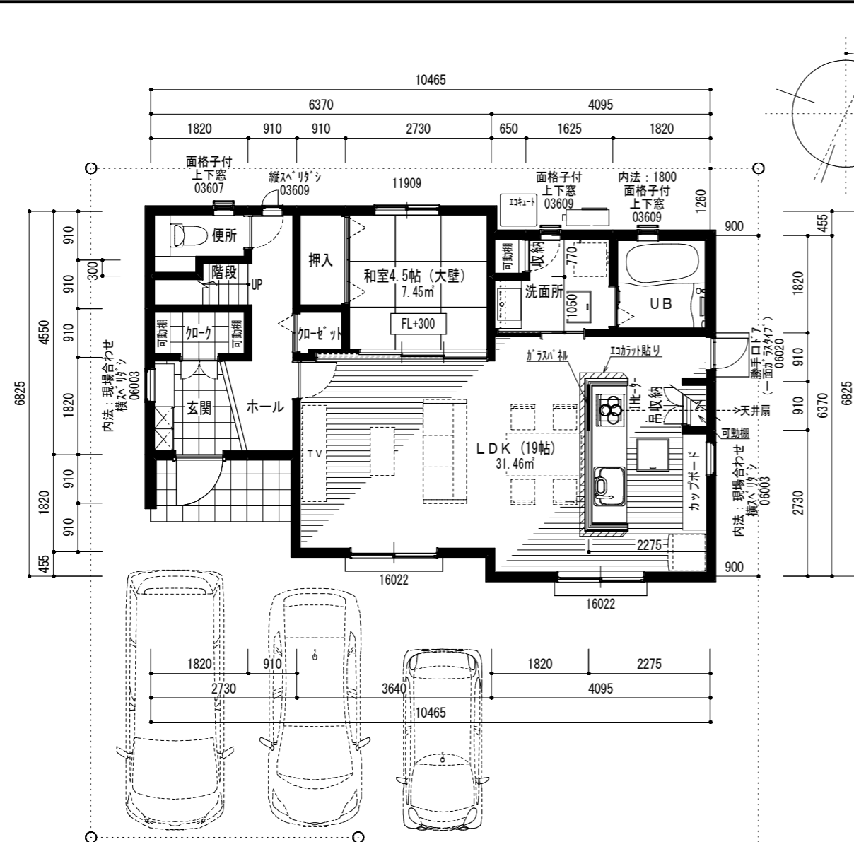
1階平面図 (プレゼン) 1/100
