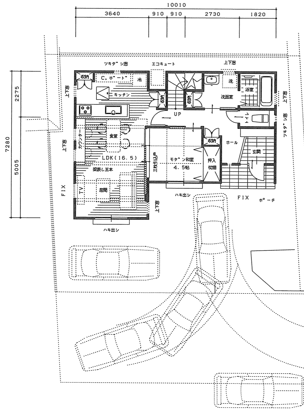
1階 平面図 1/100
