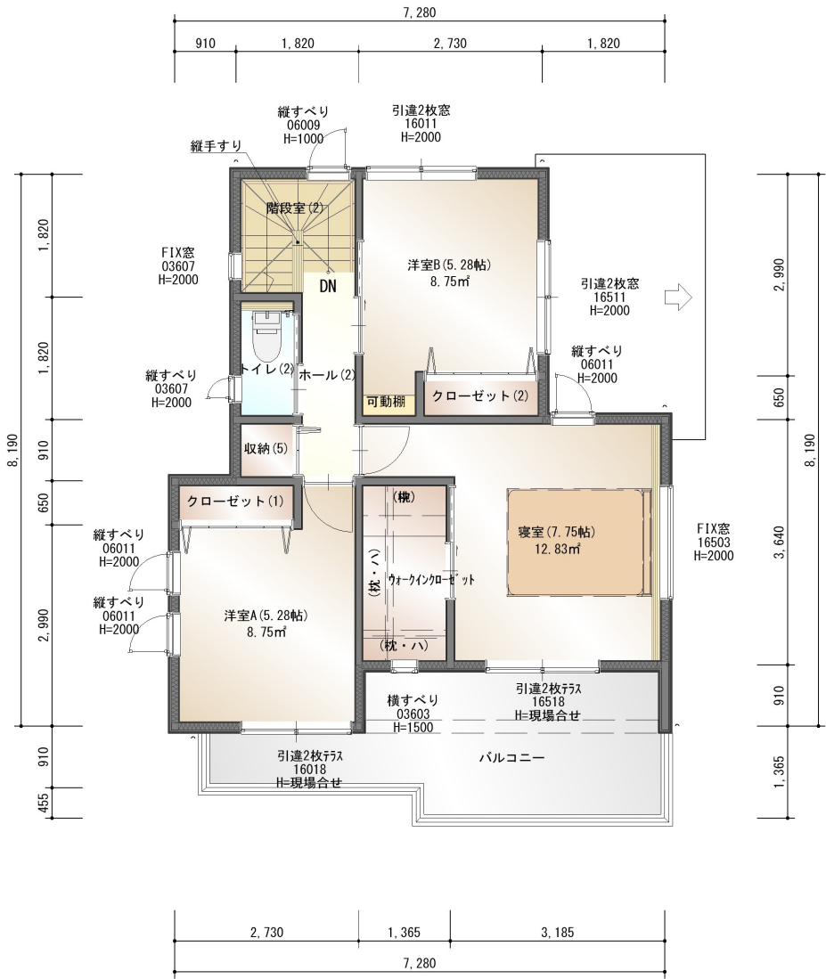
平面図
