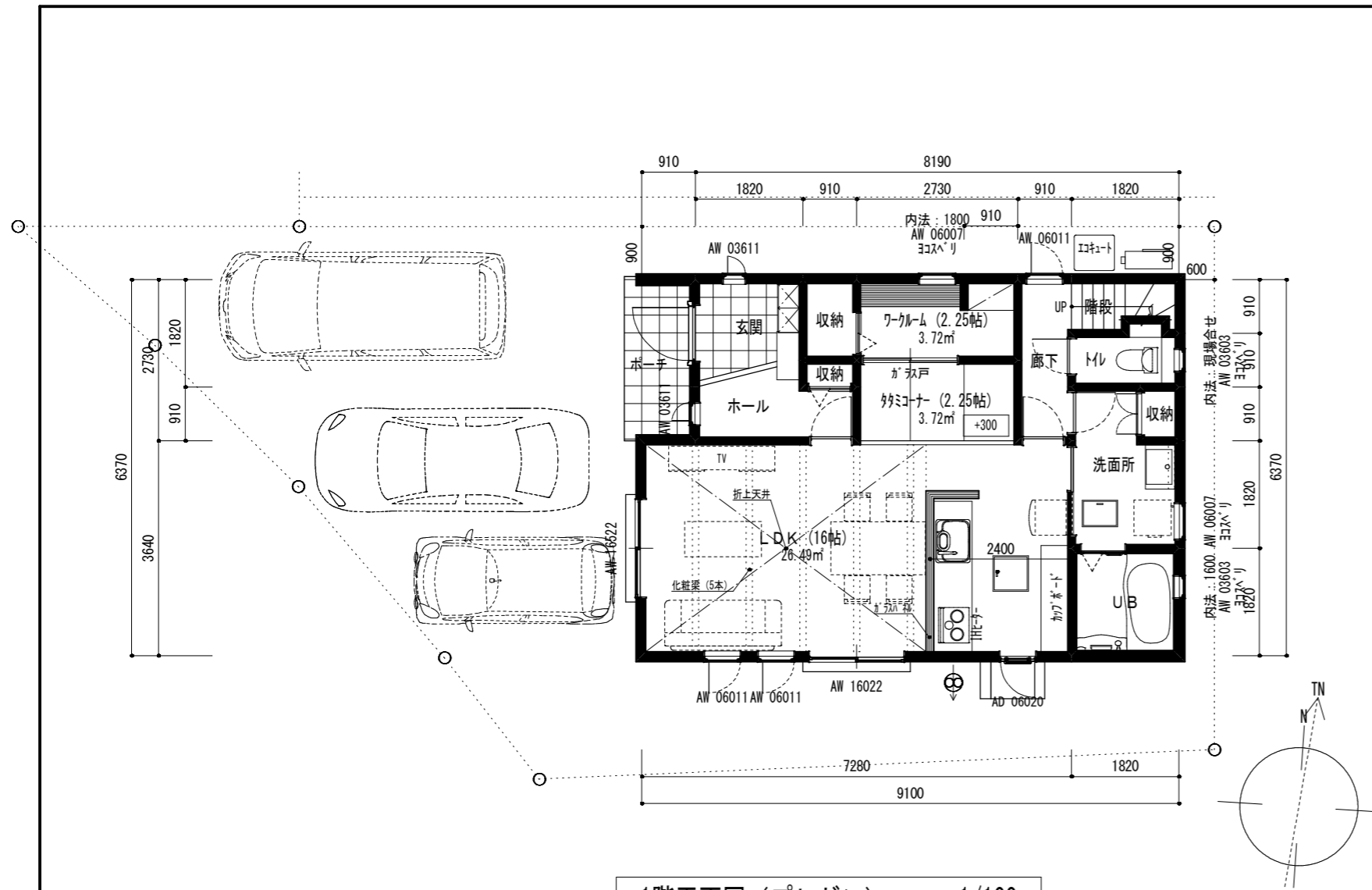
1階平面図 (プレゼン) 1/100
