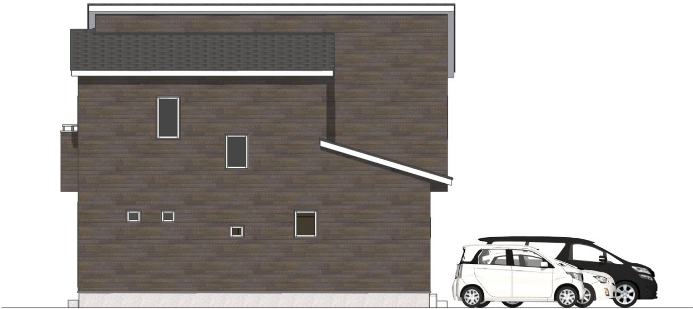
北立面図
