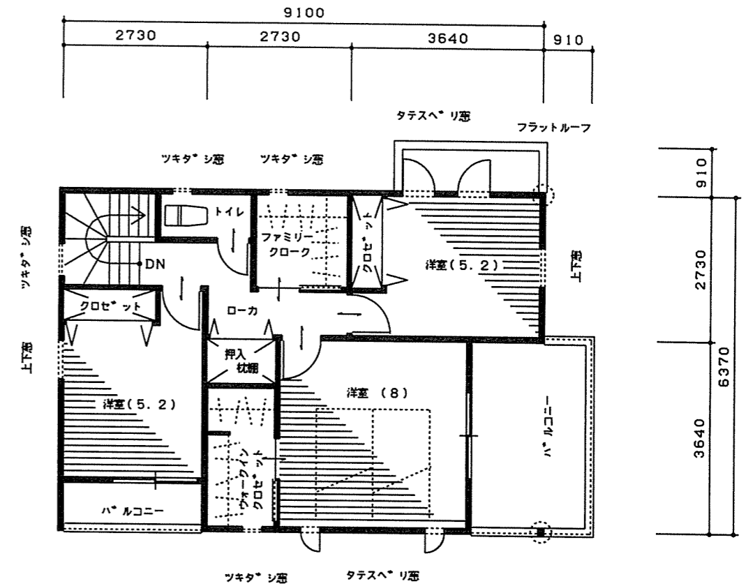
2階 平面図
