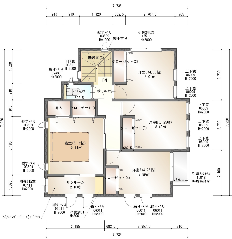
2 階平面図
