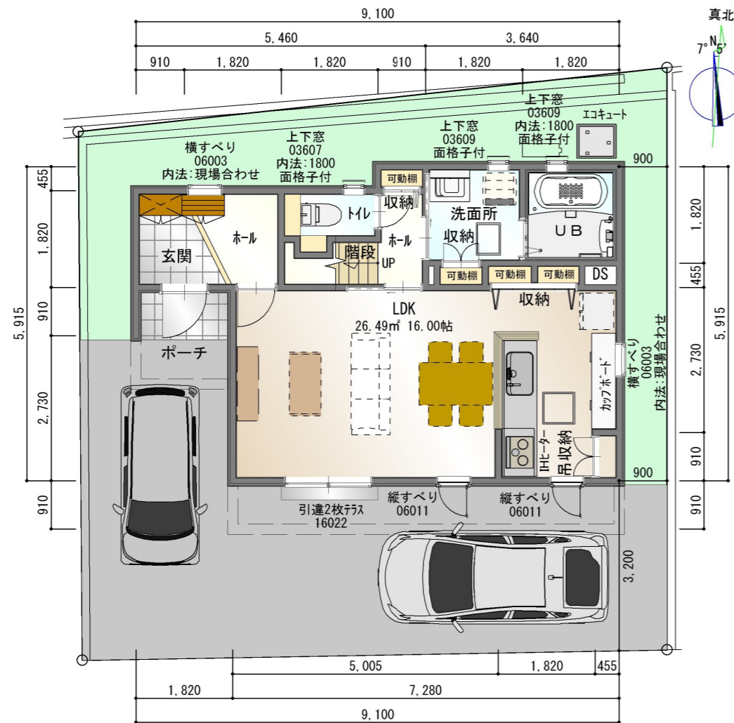
1階平面図
