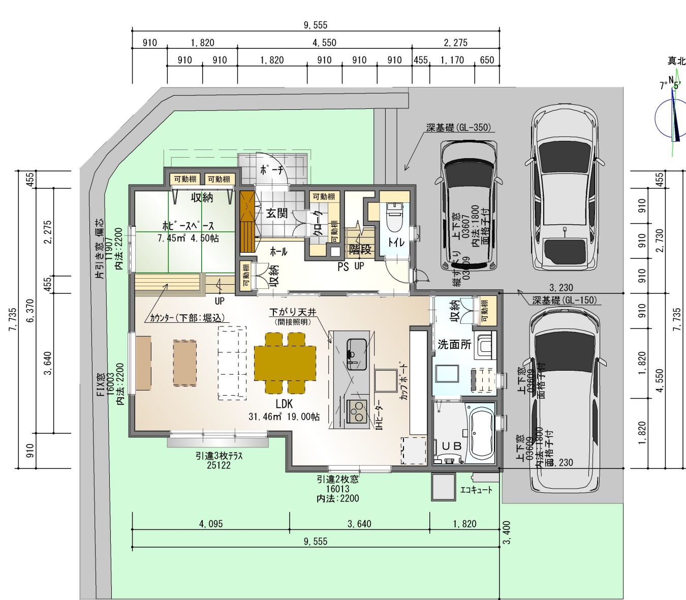
1階平面図
