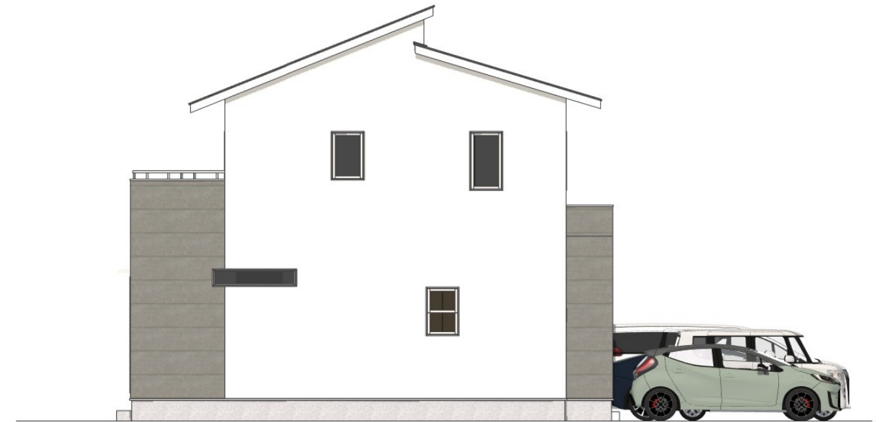
東立面図
