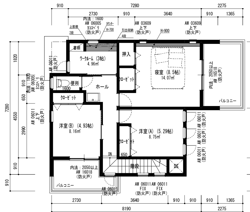
2階平面図 (プレゼン用) 1/100
