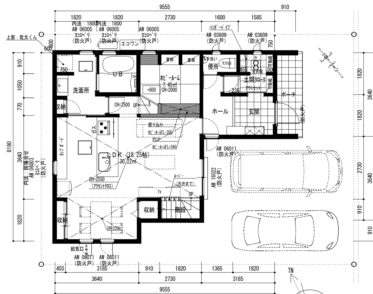
1階平面図 (プレゼン用) 1/100
