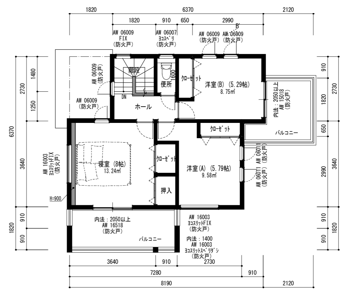
2階平面図 (プレゼン) 1/100
