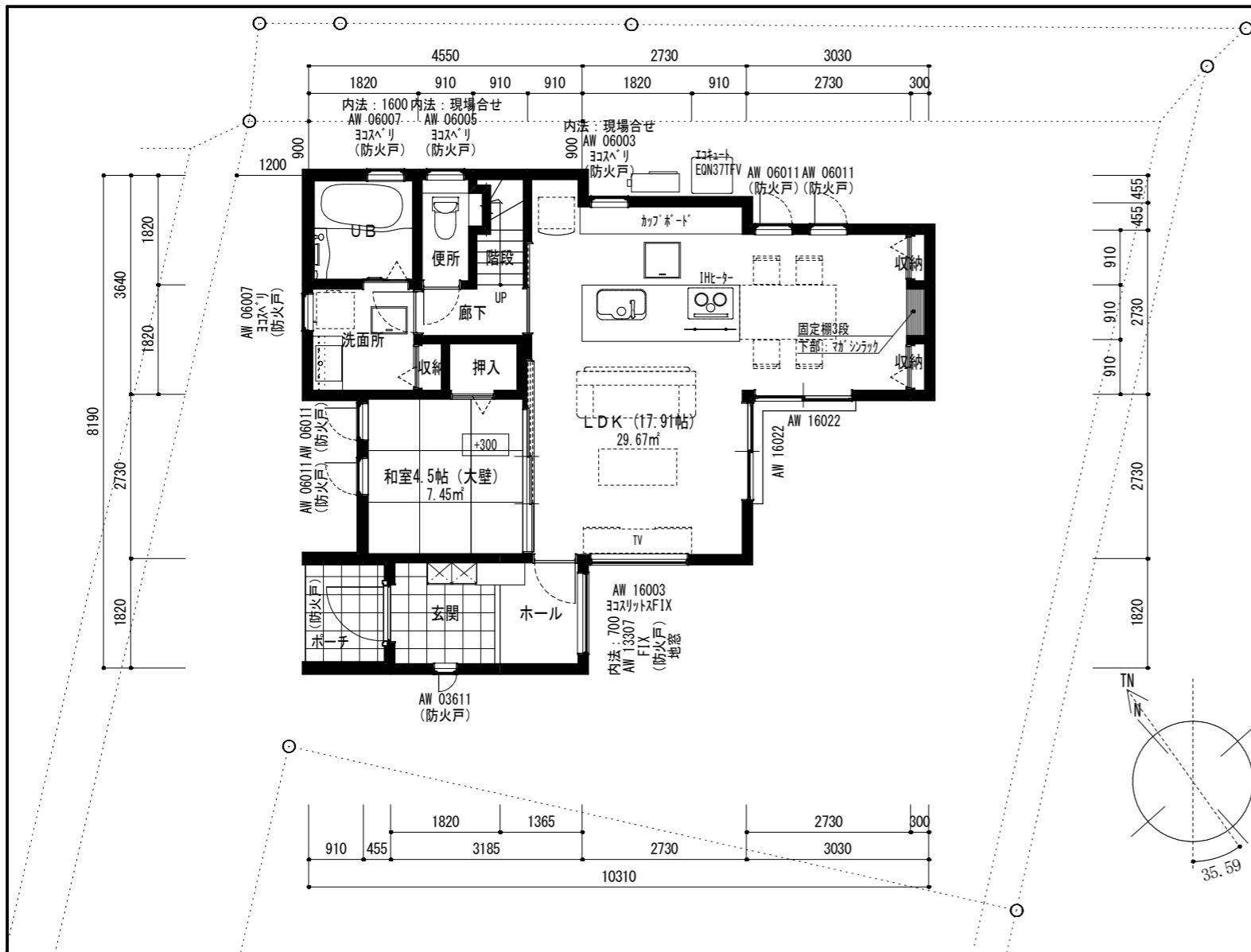
1階平面図 (プレゼン) 1/100
