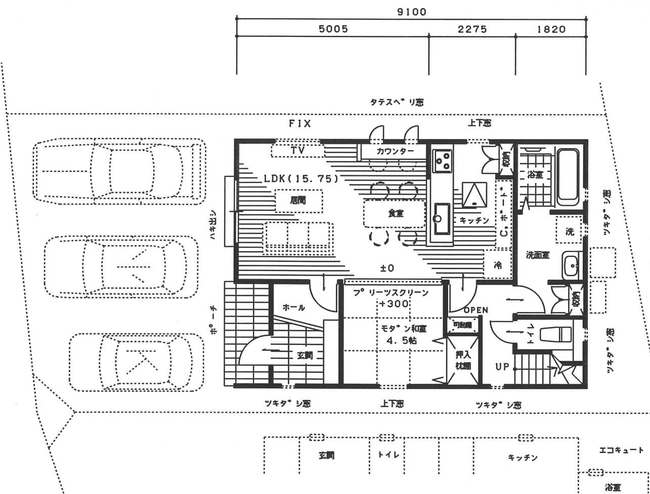
1階 平面図 1/100
