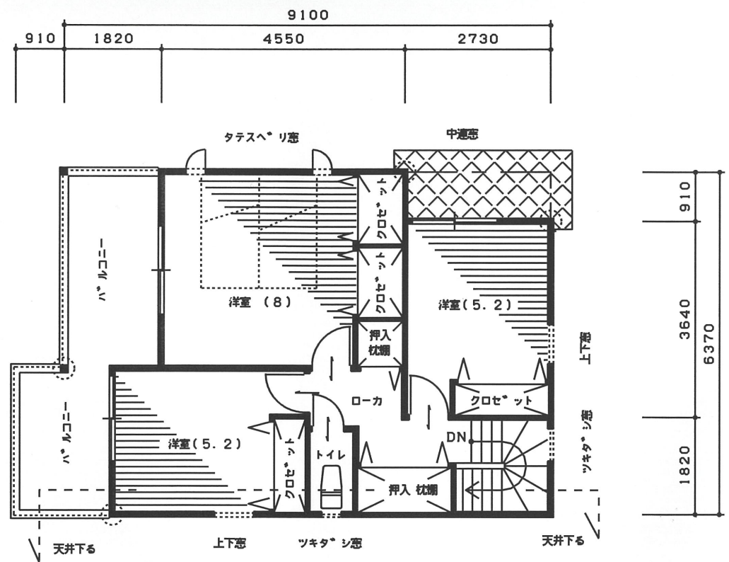
2階 平面図 1/100
