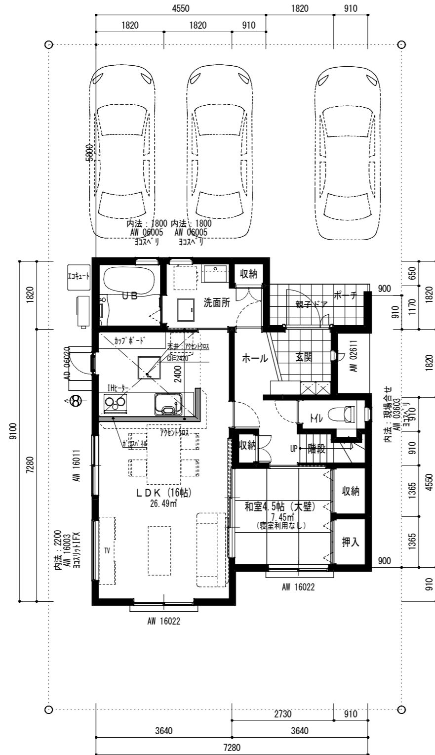
1階平面図 (プレゼン) 1/100
