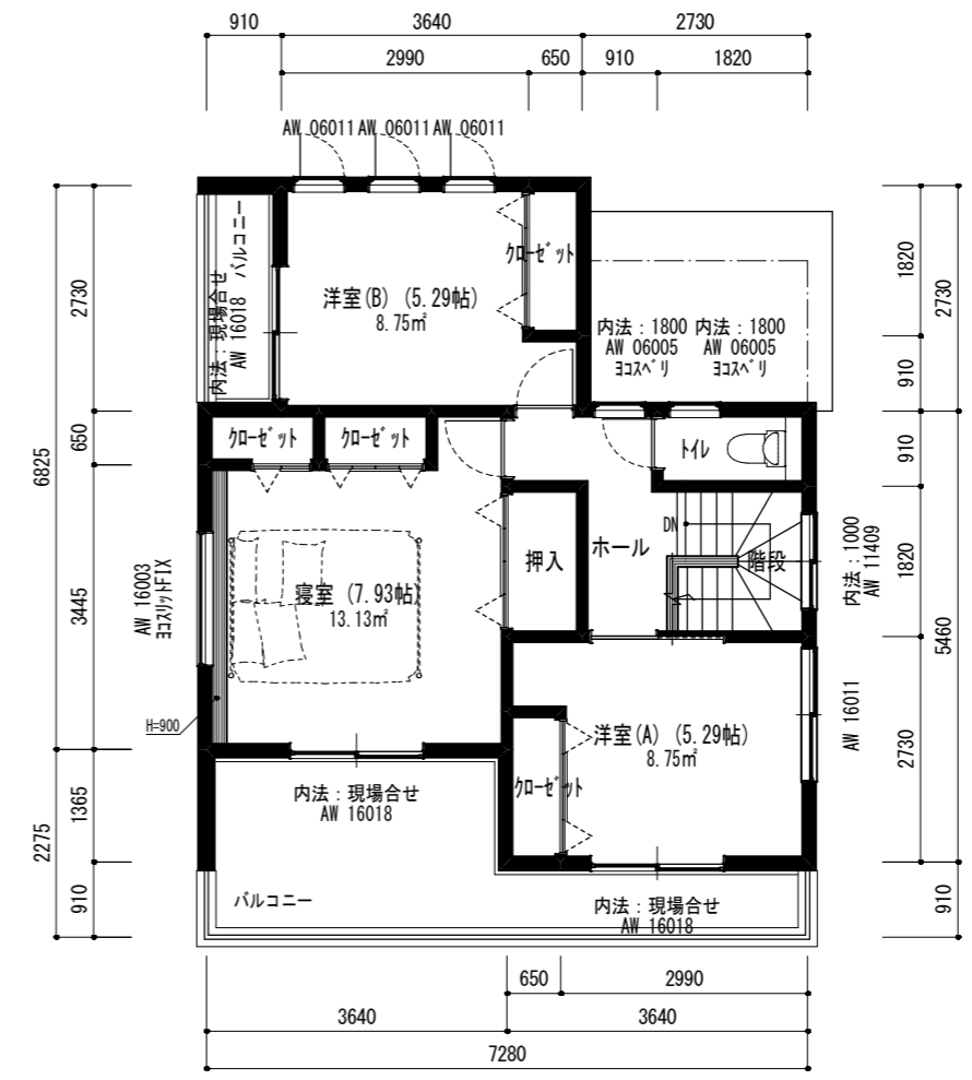
2階平面図 (プレゼン) 1/100
