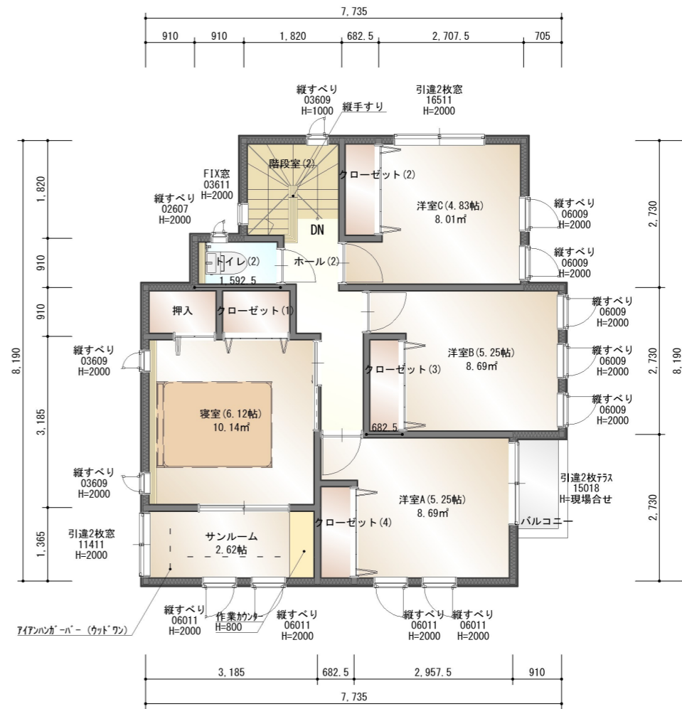
2階平面図
