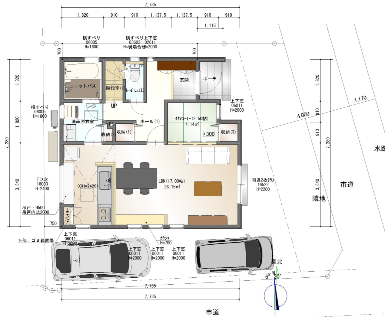
1階平面図
