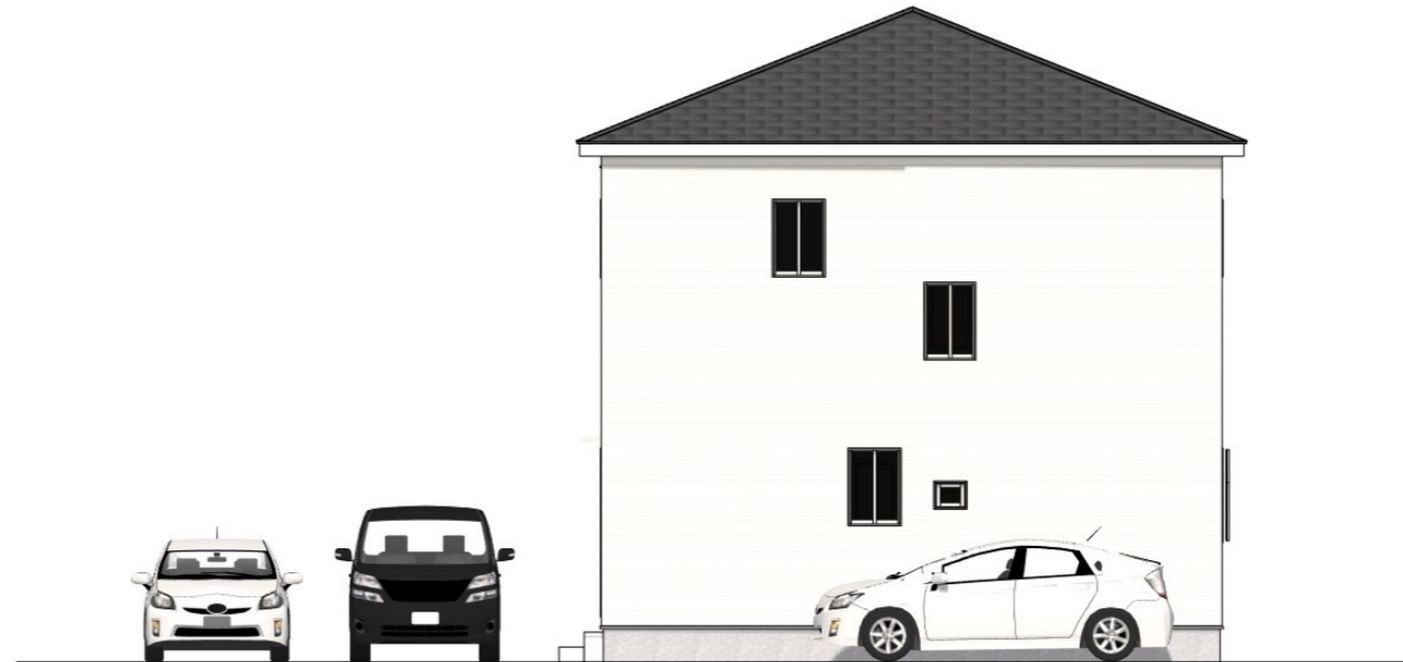
東立面図
