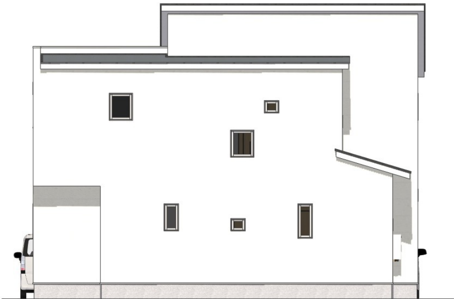
北立面図
