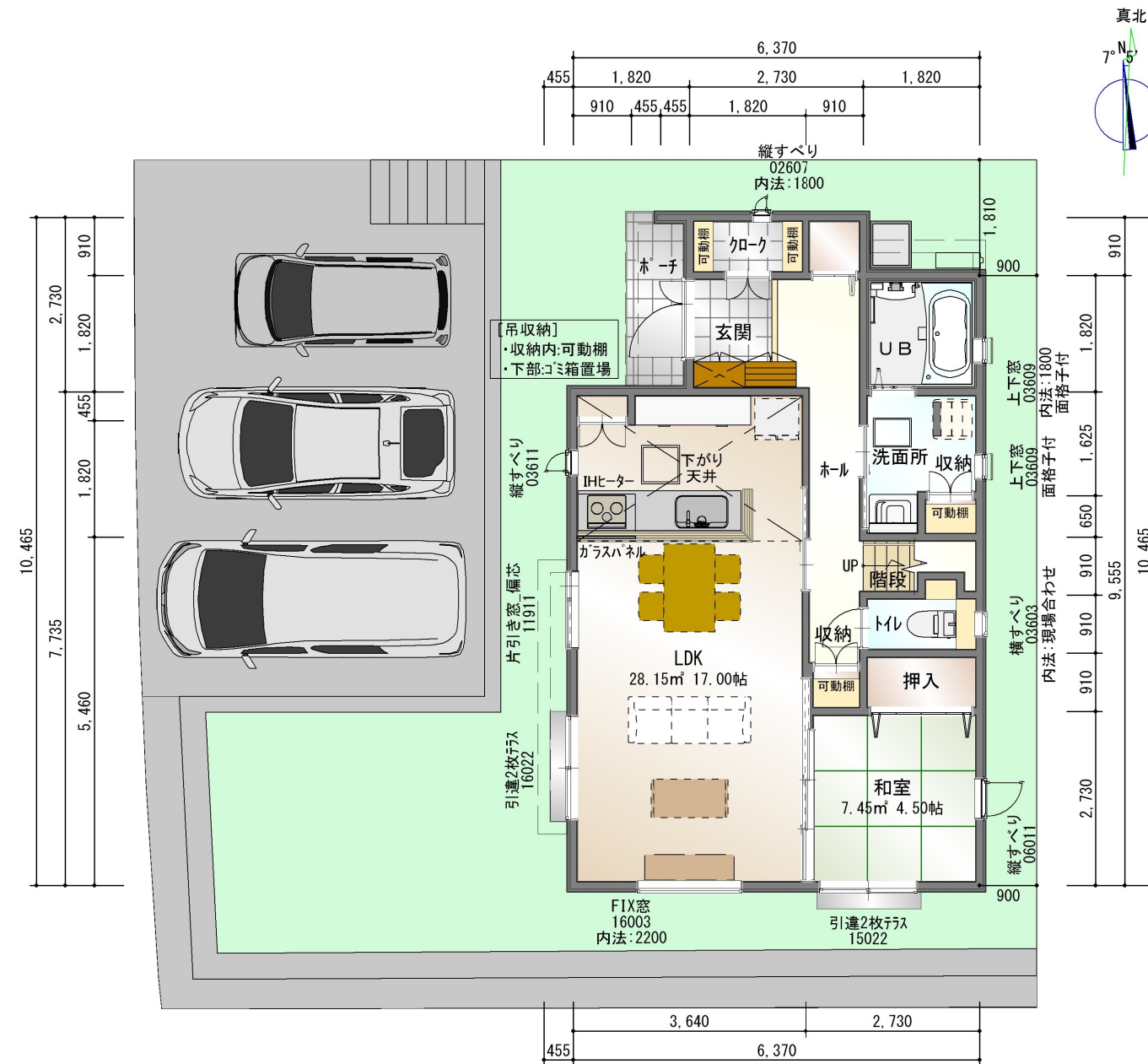
1階平面図
