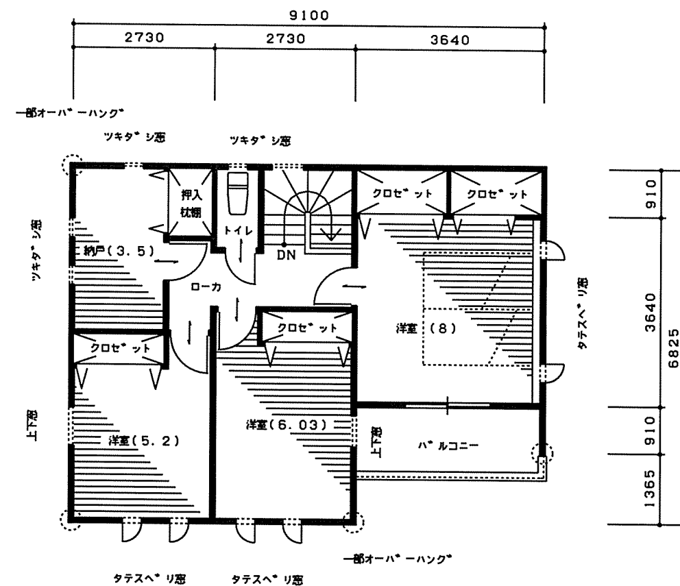
2階 平面図
