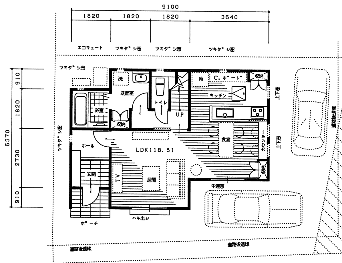
1階 平面図
