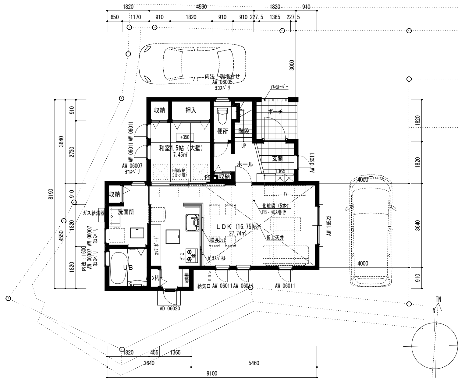
1階平面図 (プレゼン用) 1/100
