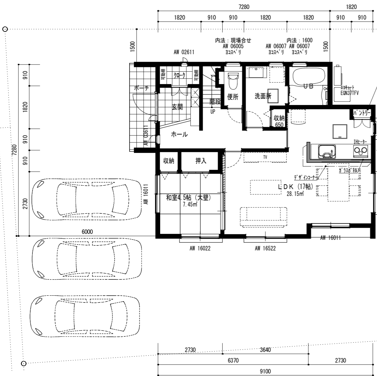
1階平面図 (プレゼン用) 1/100
