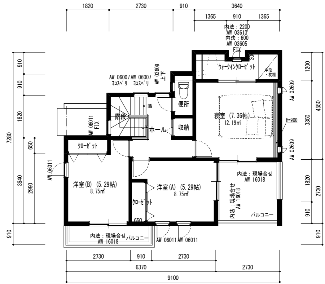
2階平面図 (プレゼン用) 1/100
