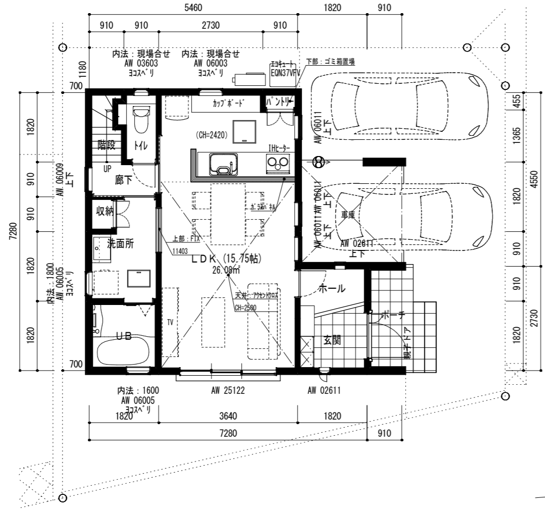
1階平面図 (プレゼン) 1/100
