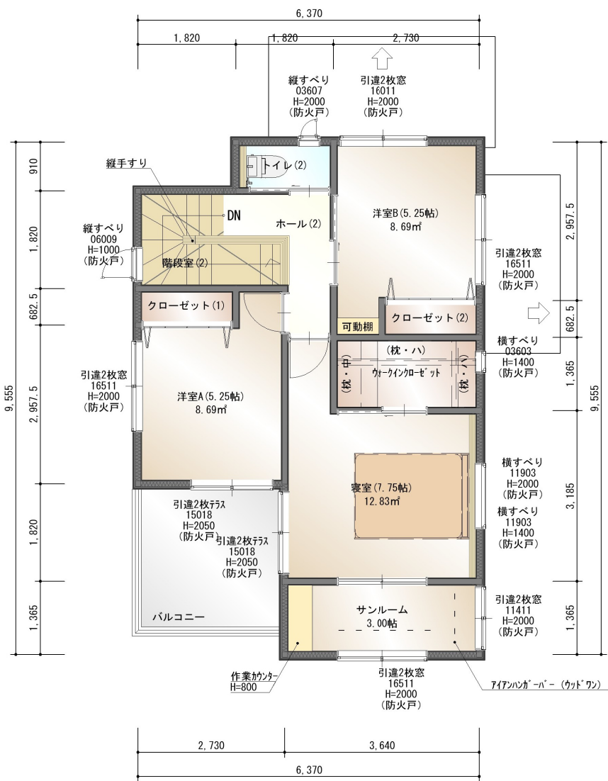
2 階平面図
