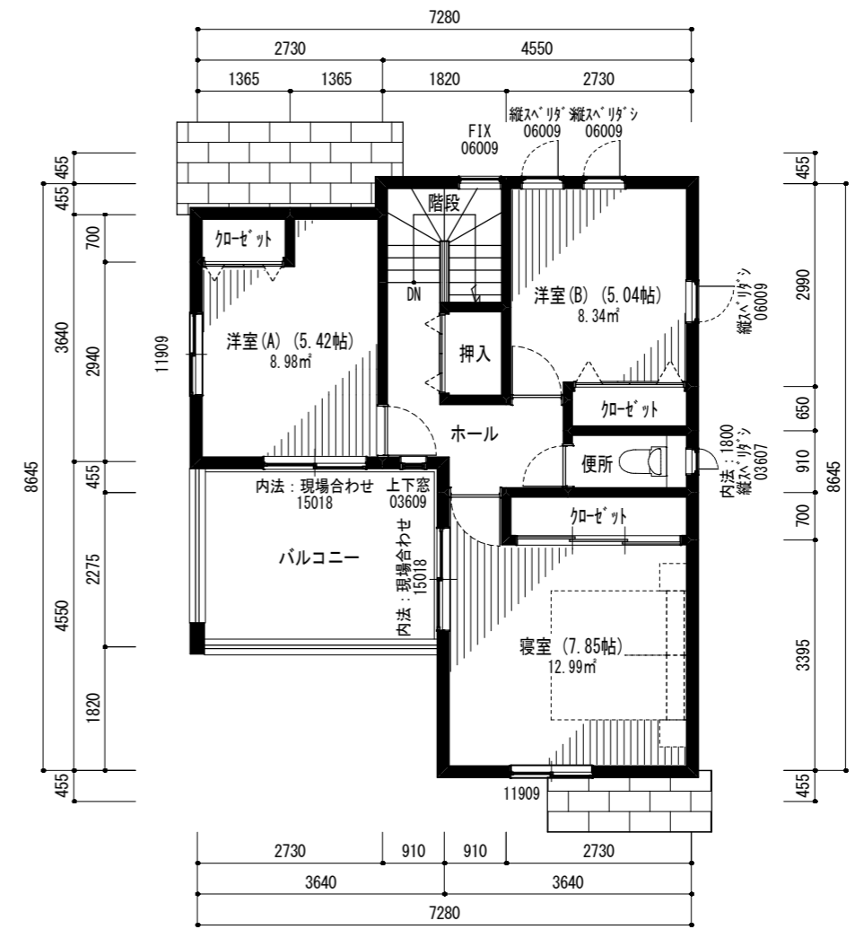
2階平面図 (プレゼン) 1/100
