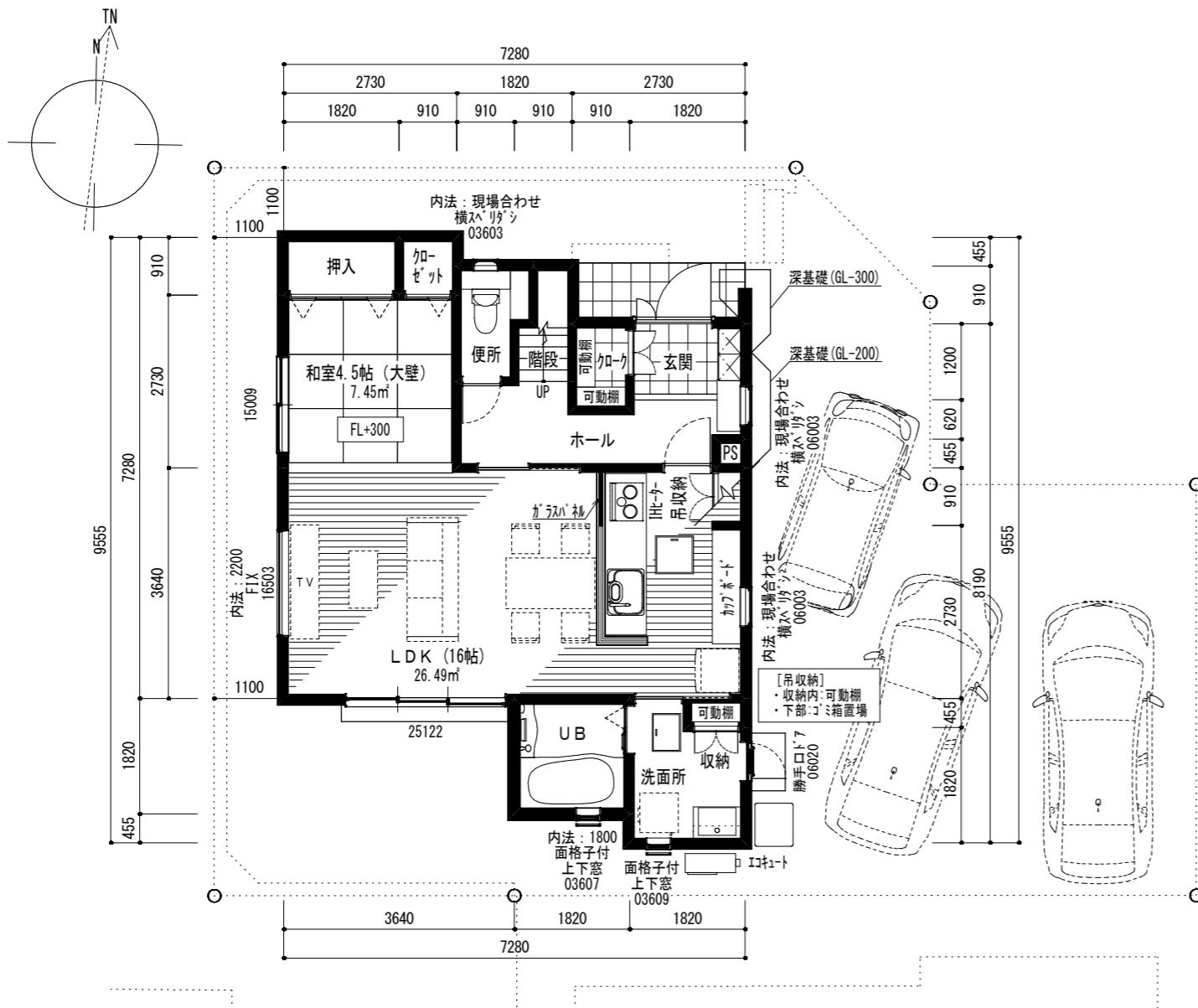
1階平面図 (プレゼン) 1/100
