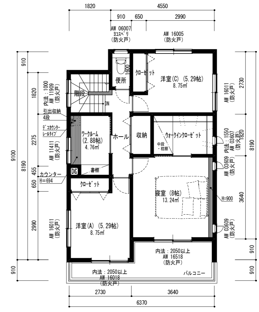
2階平面図 (プレゼン用) 1/100
