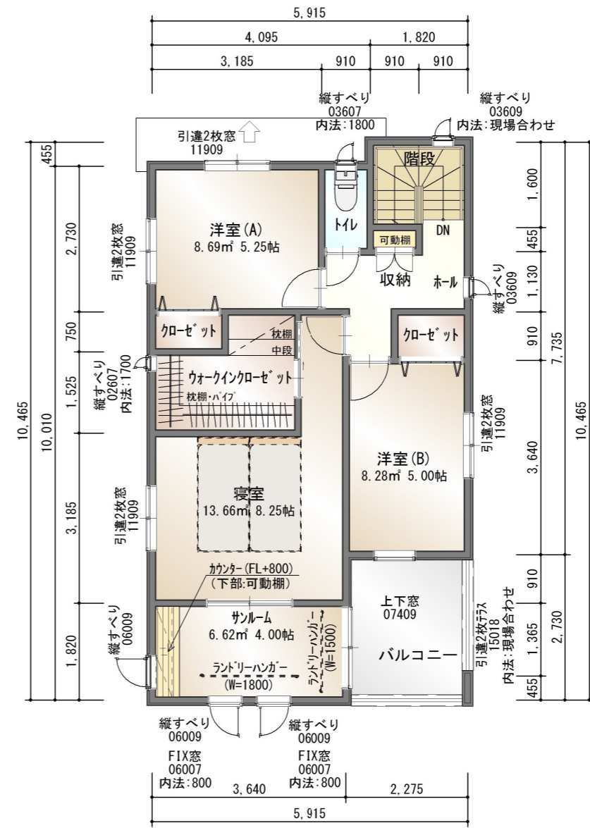
2階平面図
