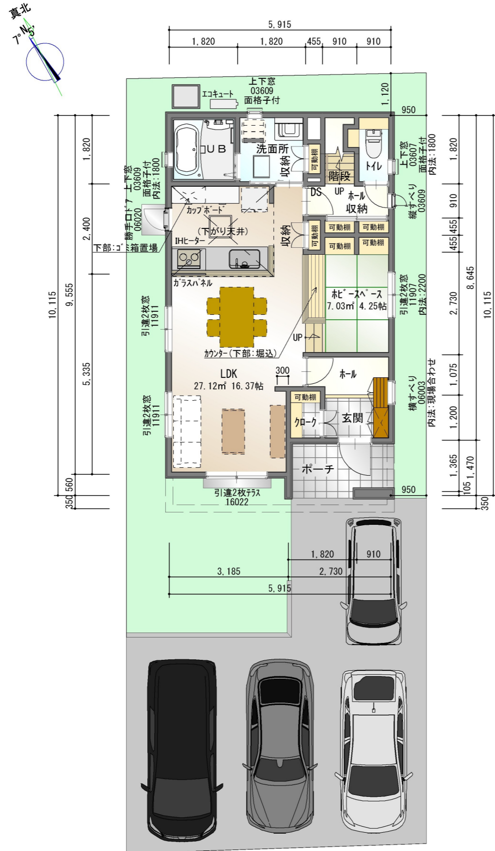
1階平面図
