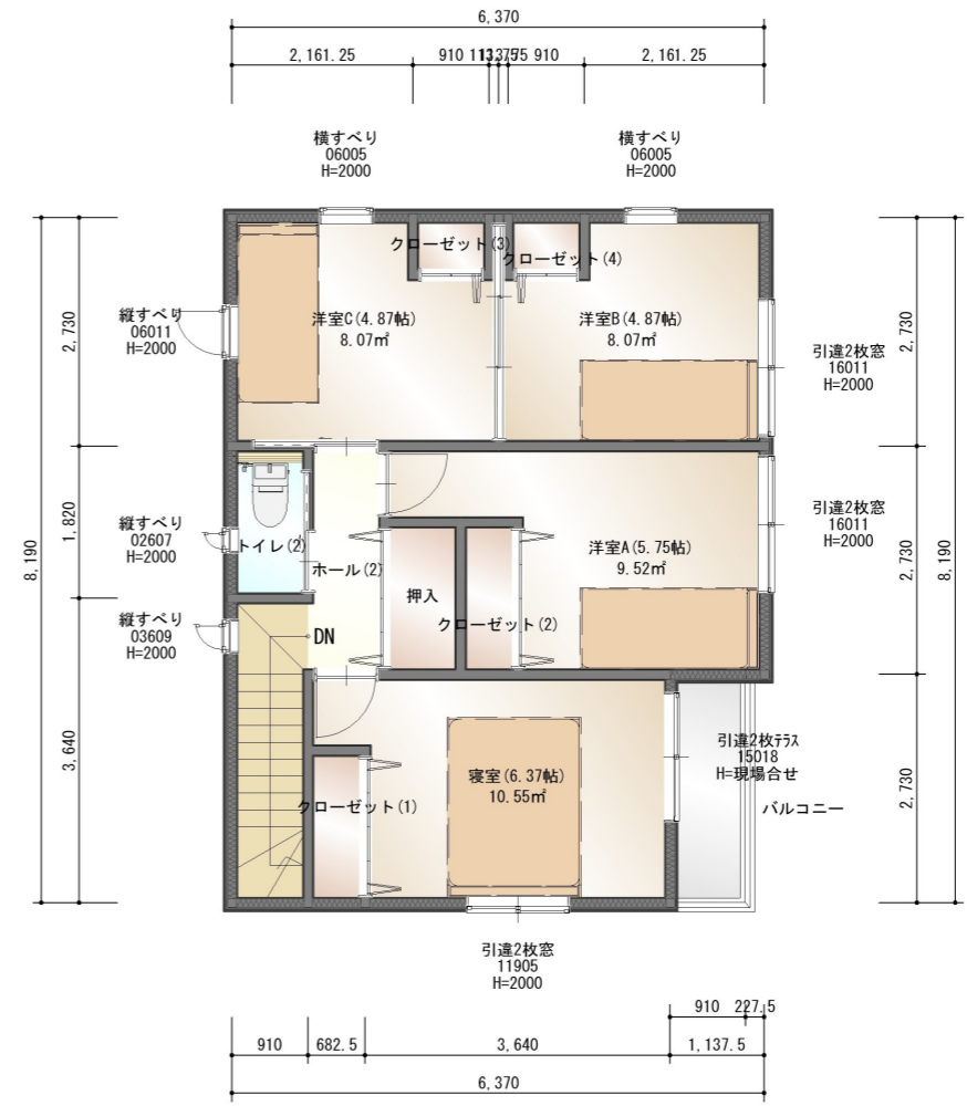
2階平面図
