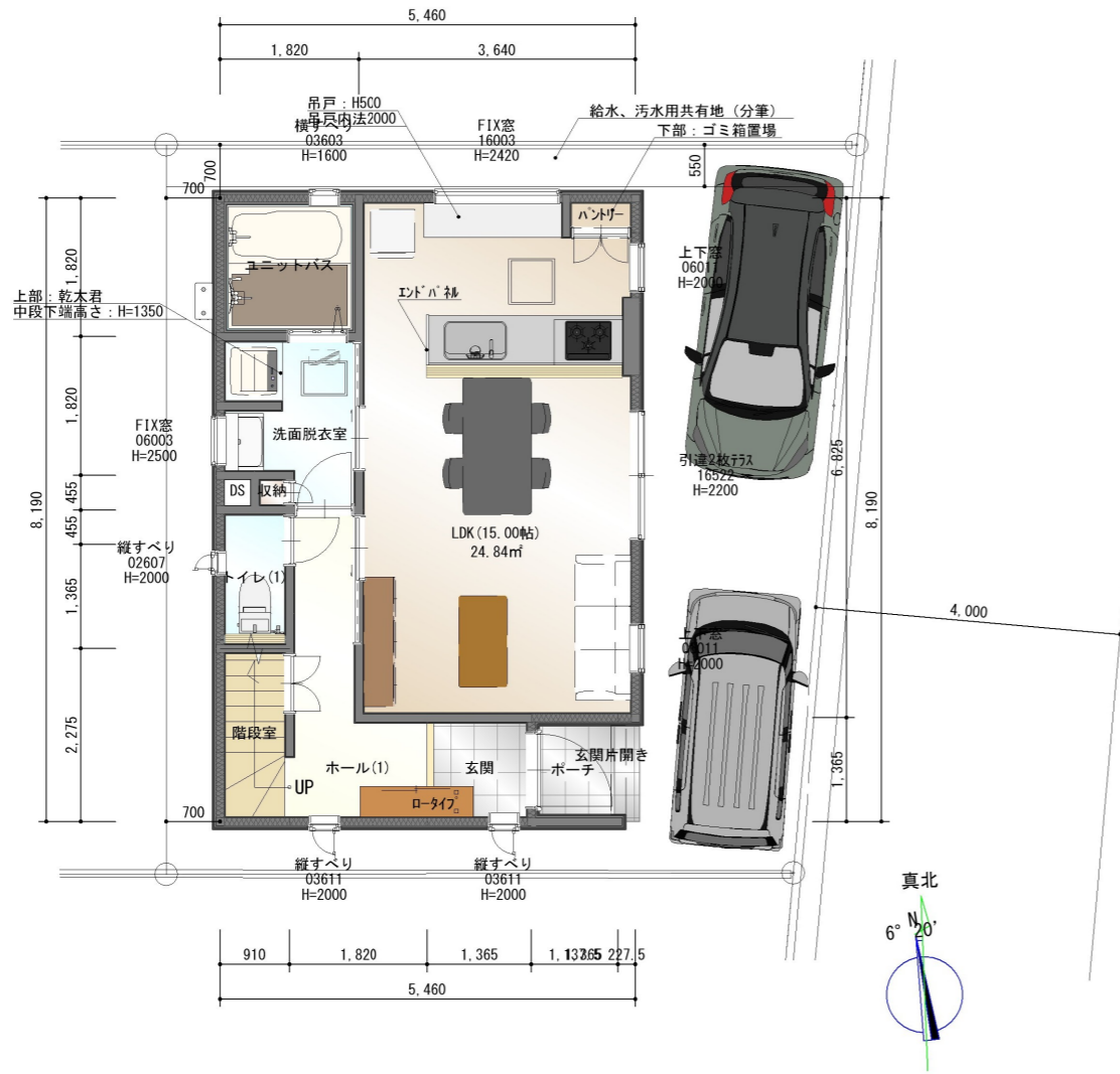
1階平面図
