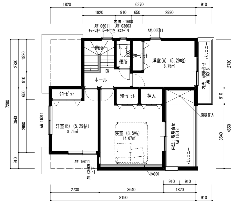
2階平面図 (プレゼン用) 1/100
