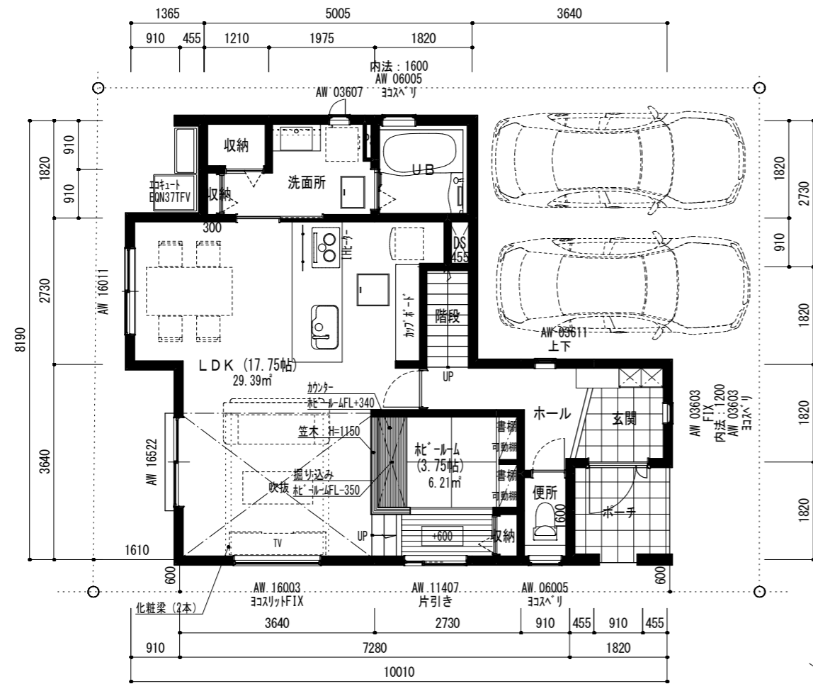
1階平面図 (プレゼン) 1/100
