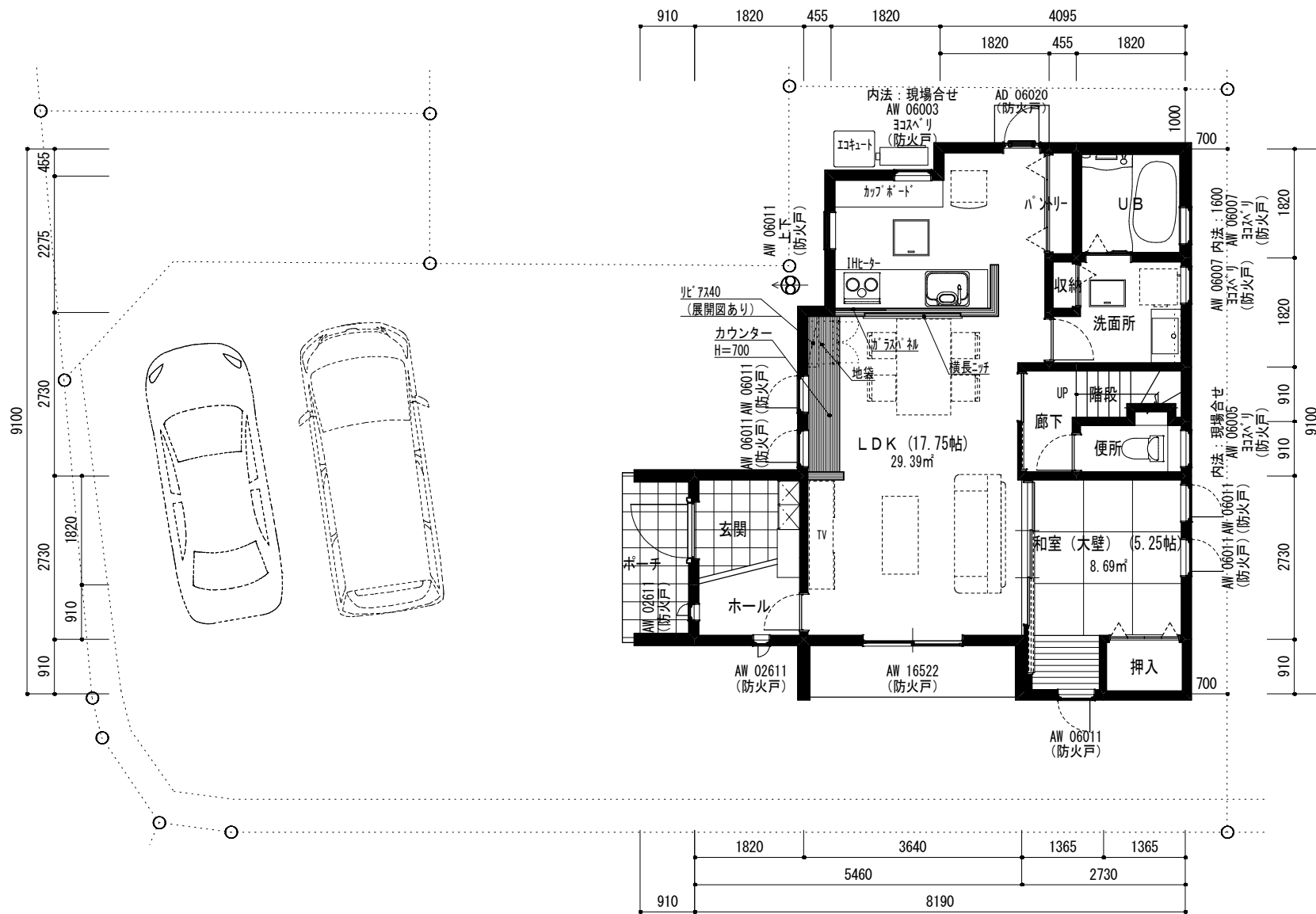
1階平面図 (プレゼン) 1/100
