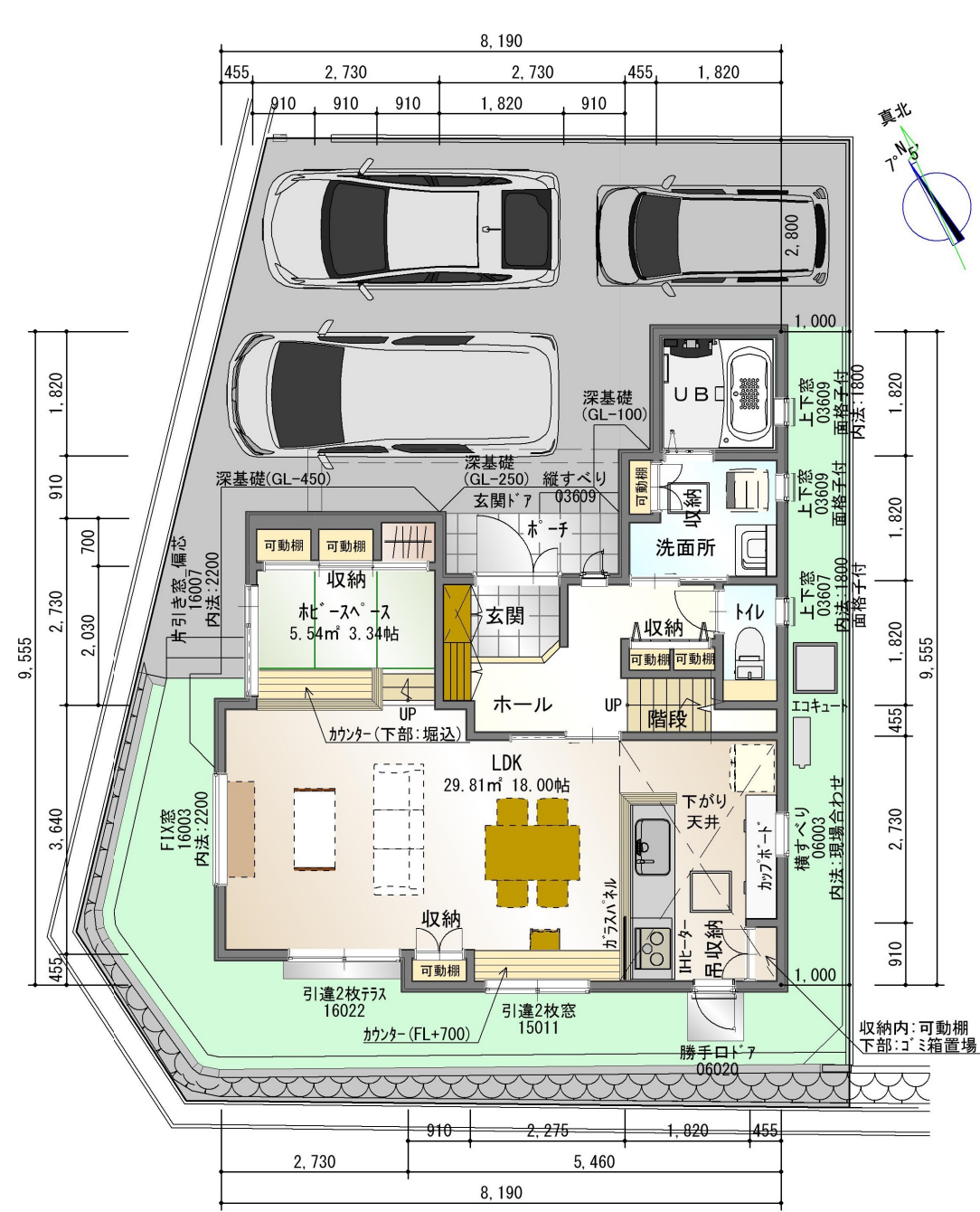
1階平面図
