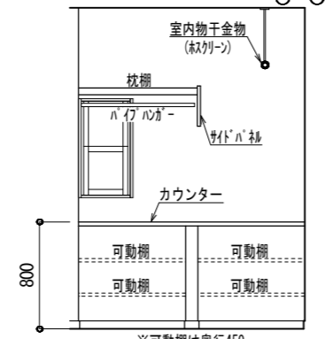
洗面所展開図 1/50
