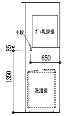
ガス乾燥機スペース断面図 1/50
