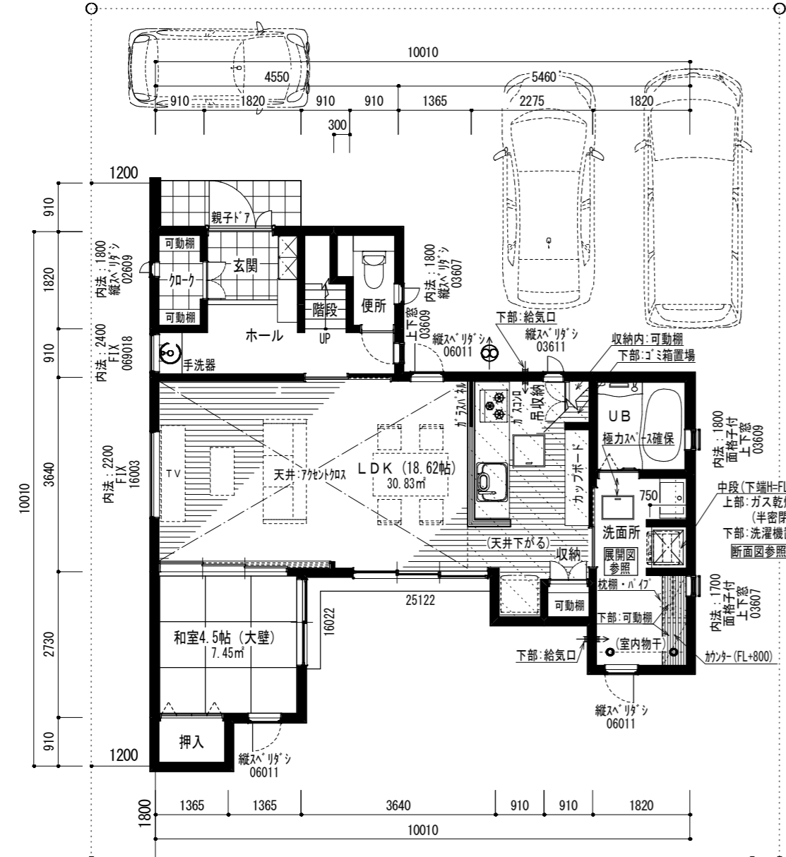
1階平面図 (プレゼン) 1/100
