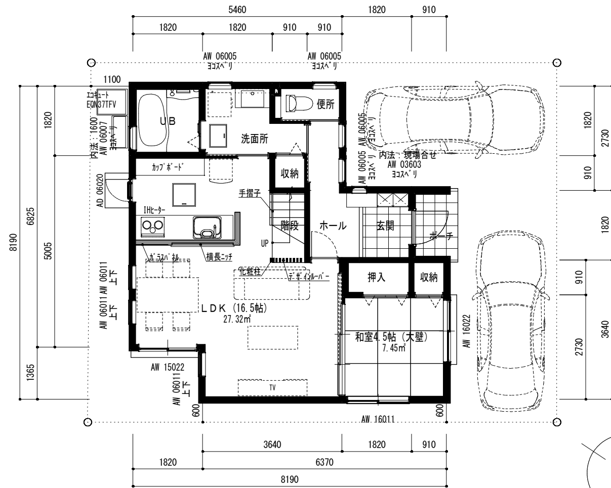
1階平面図 (プレゼン) 1/100
