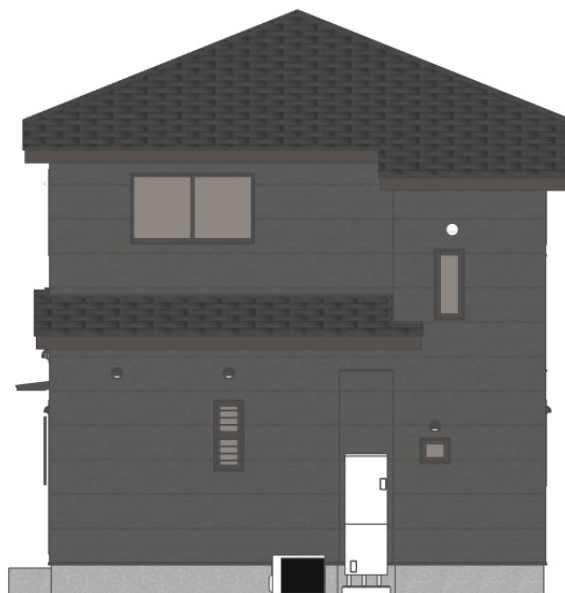
北立面图
