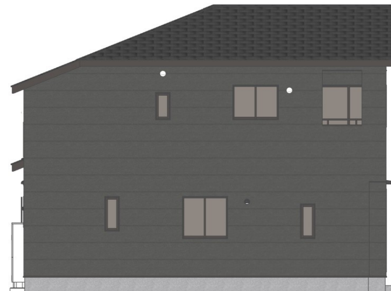
西立面图
