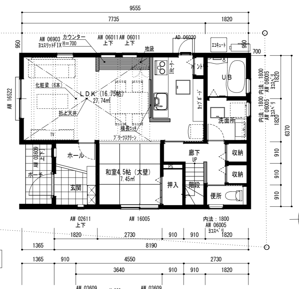
1階平面図 (プレゼン用) 1/100
