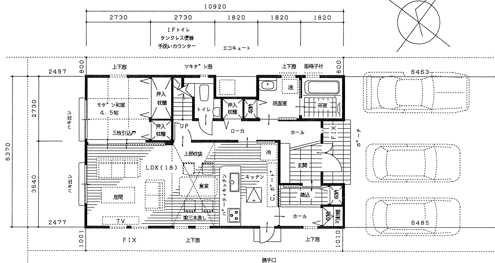
1階 平面図
