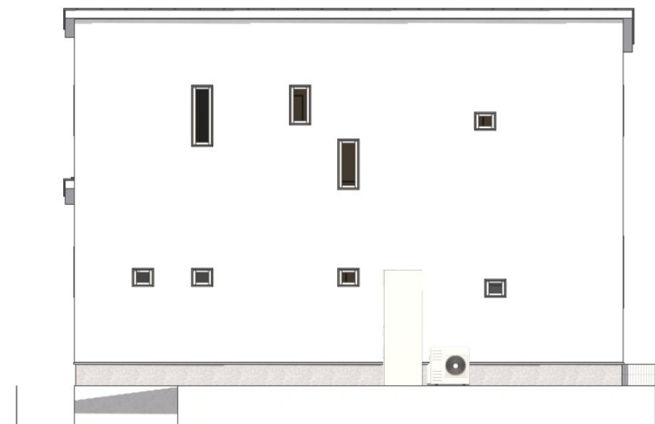
西立面図
