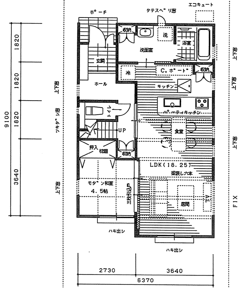
1階 平面図 1/100
