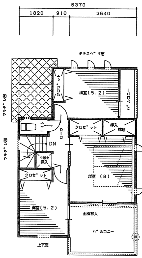
2階 平面図 1/100
