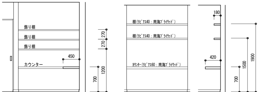
LDKカウンター展開図 1/50
