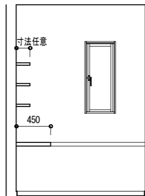
LDKカウンター展開図 1/50
