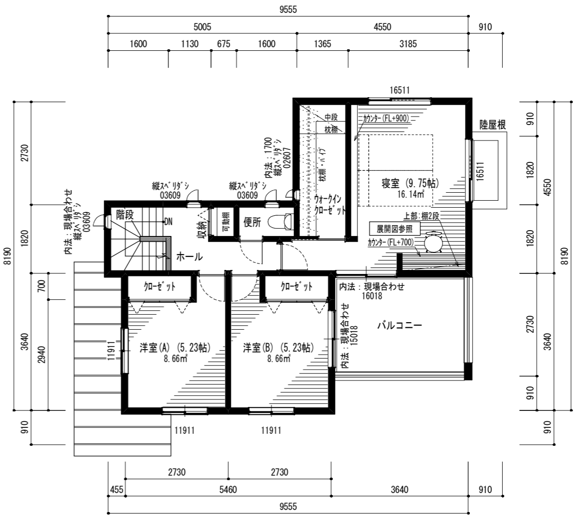
2階平面図 (プレゼン) 1/100
