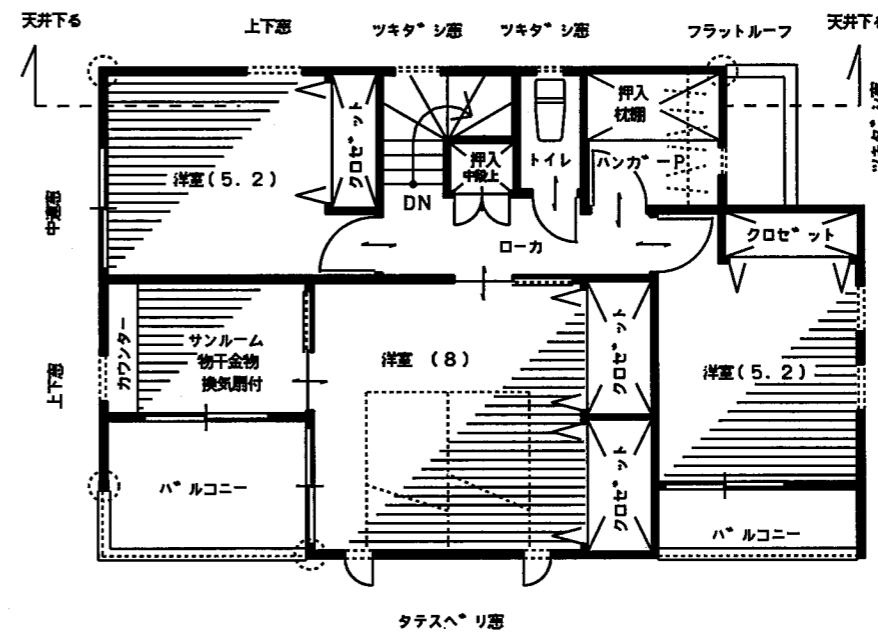
2階 平面図
