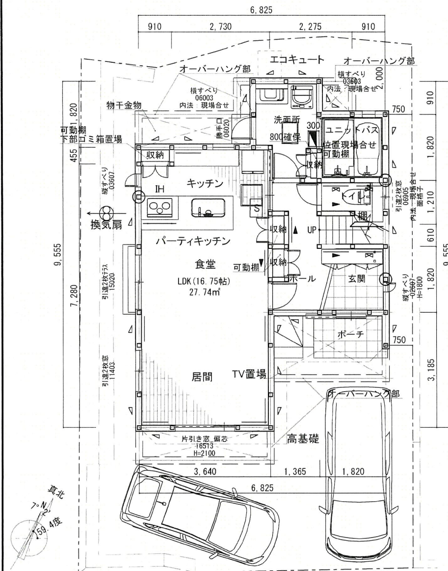
配置図兼1階平面図1/100
