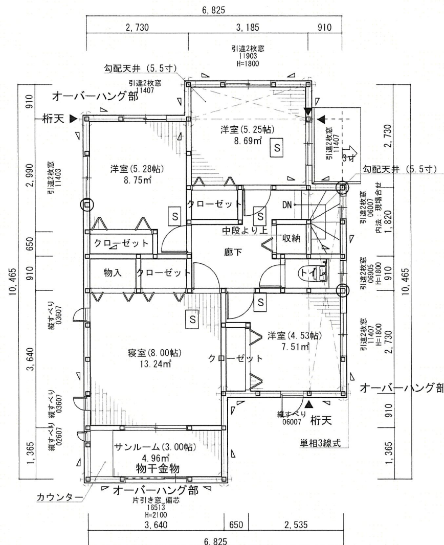
2階平面図1/100
