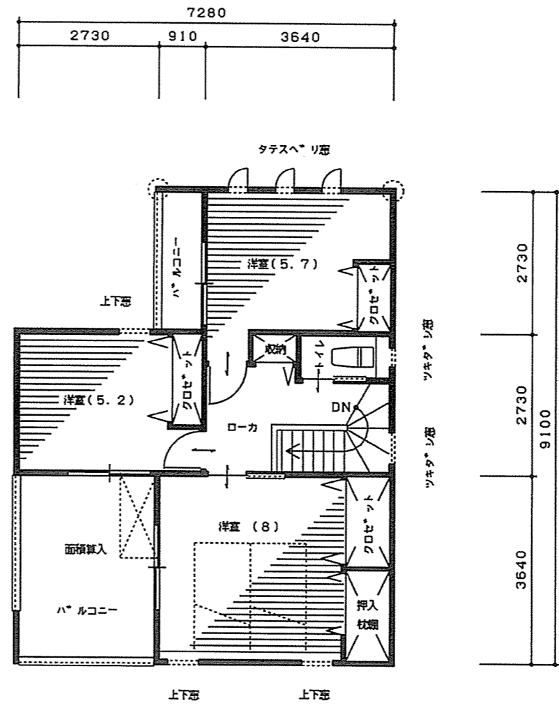
2階 平面図 1/100
