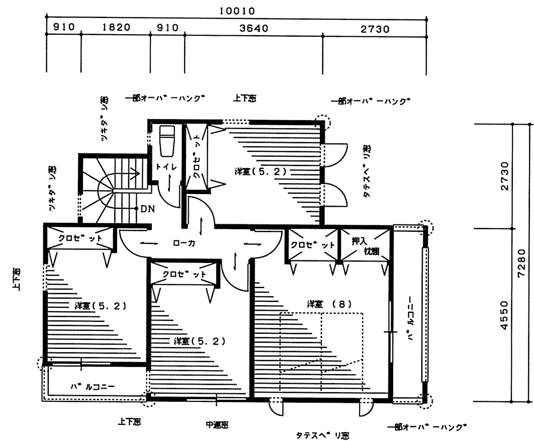
2階 平面図
