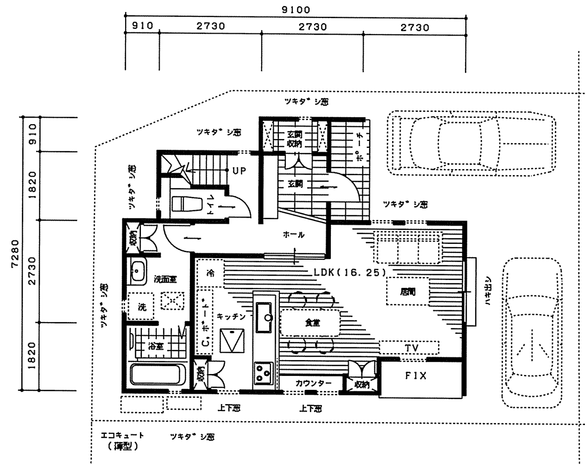
1階 平面図
