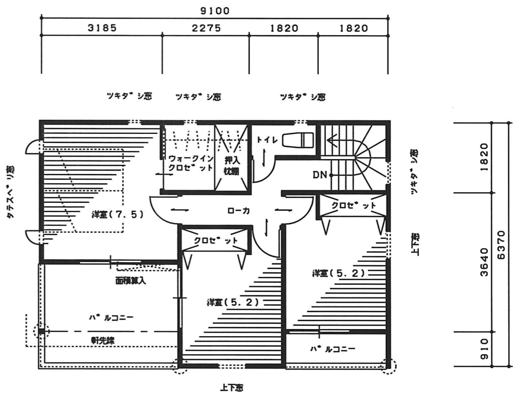
2階 平面図
