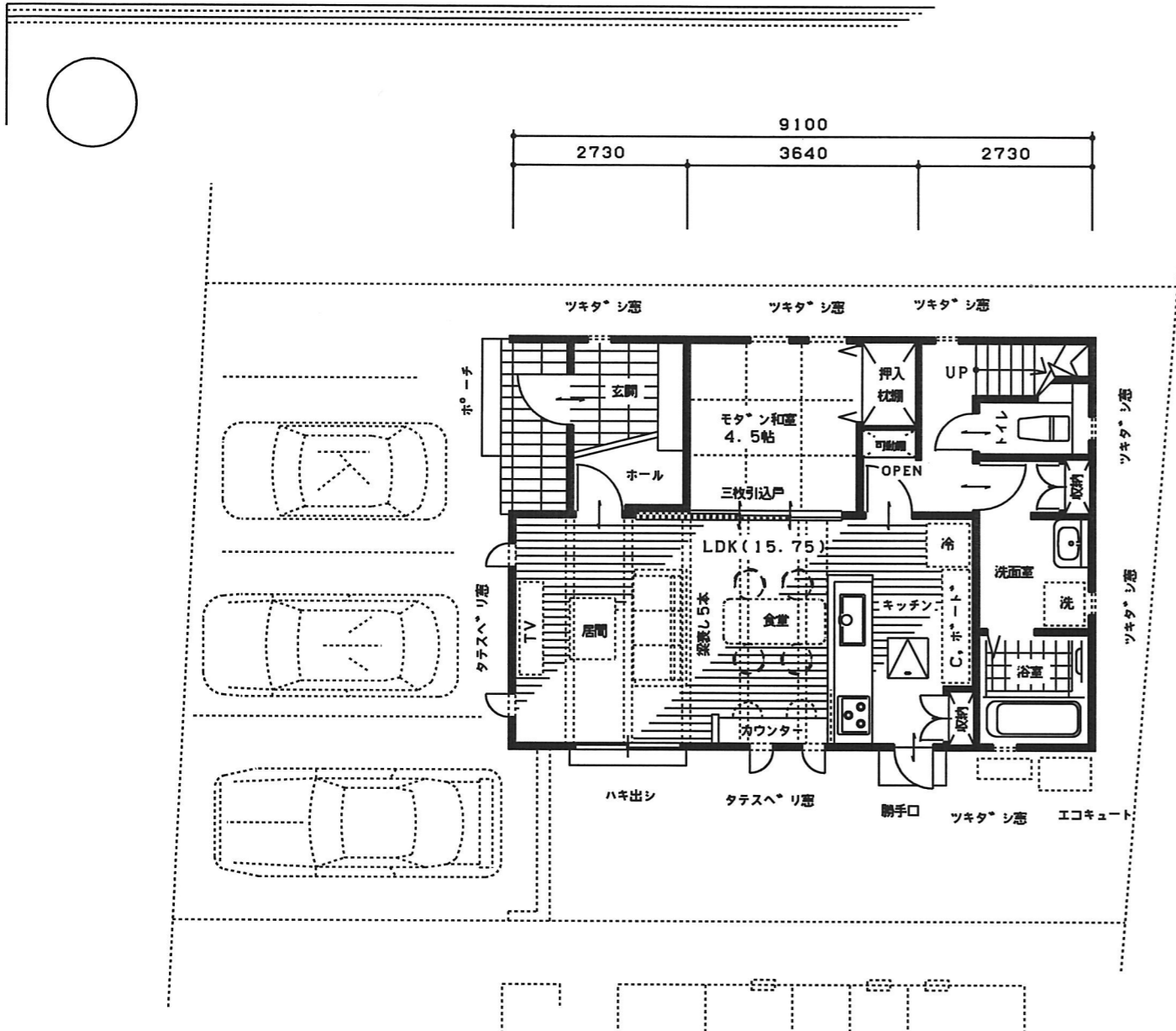
1階 平面図
